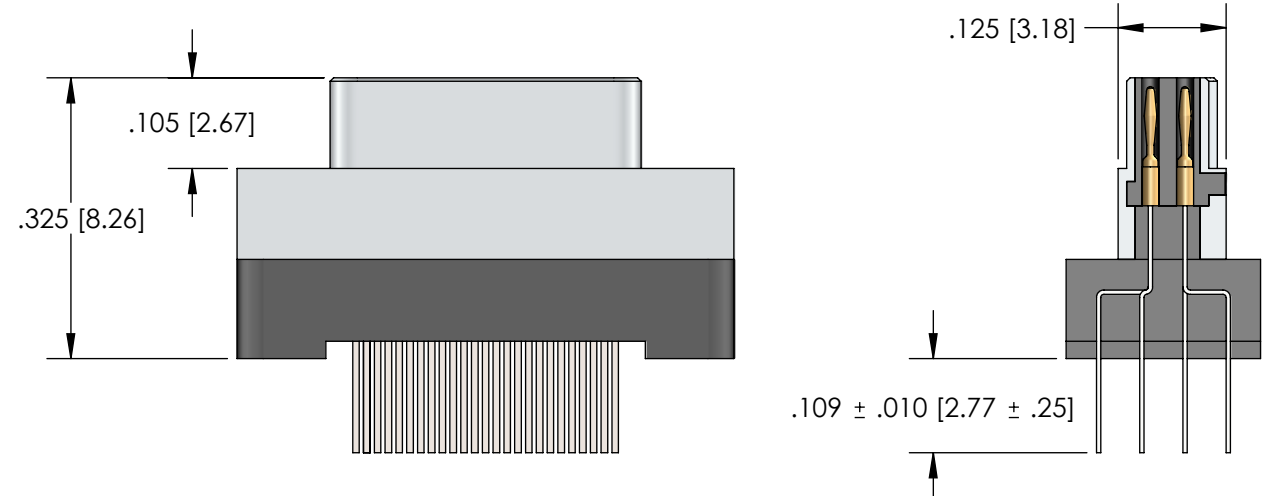
PLUG (PINS)
